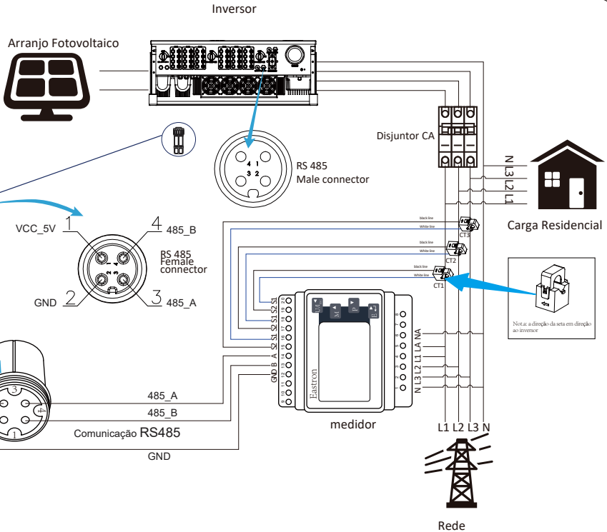
Figura 7.13 Diagrama da Comunicação do medidor Eastron
