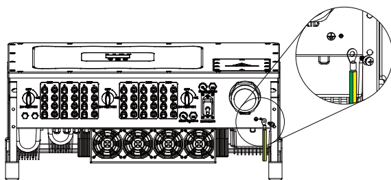
Figura 5.12 A instalação do Aterramento da Carcaça
