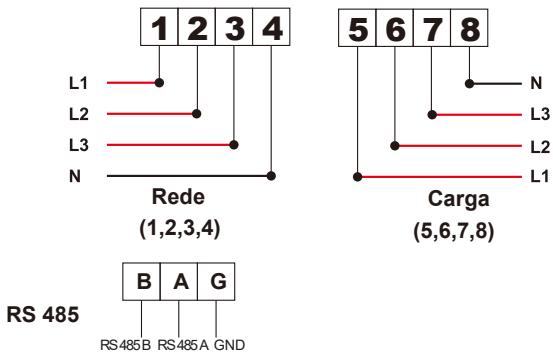
Figura 7.10 Medidor Eastron
